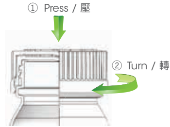
兒童安全瓶 Child-Resistant Bottle
